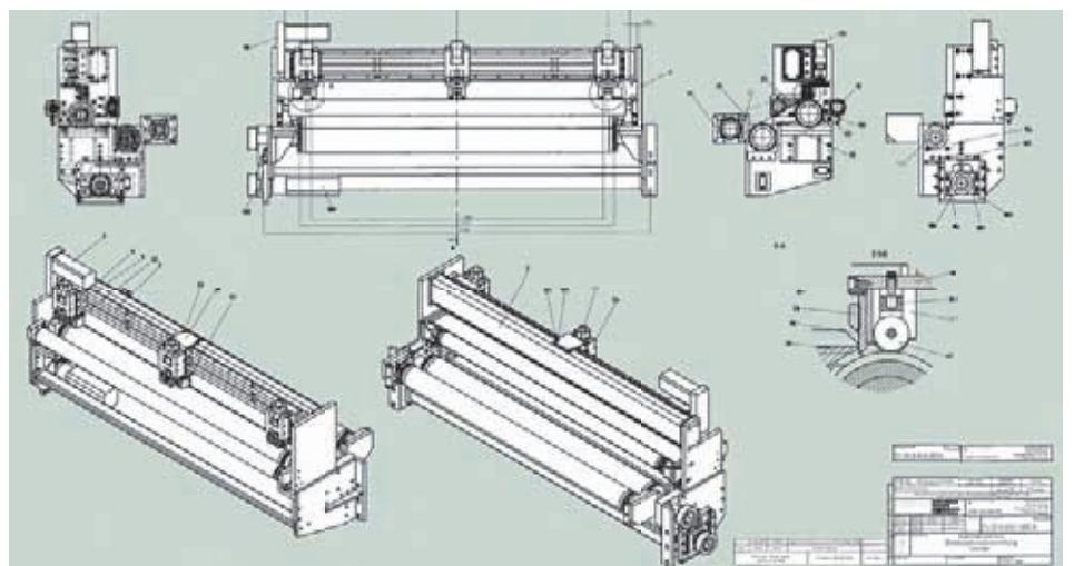
Zusammenbau Streifeneinschneidvorrichtung
