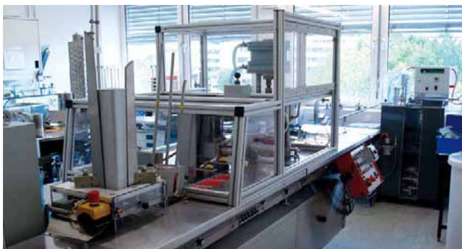
Siegelmaschine für die Pharmakonfektionierung u.a. mit komplett nachgerüsteten Sicherheitskomponenten
